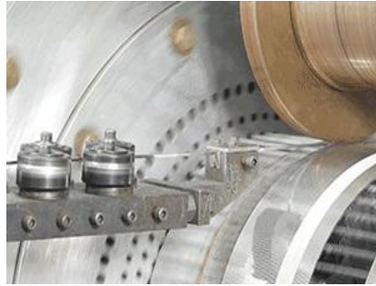
Wire rolling
